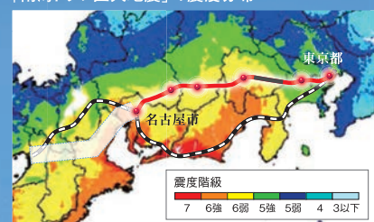
「南海トラフ巨大地震」の震度分布
